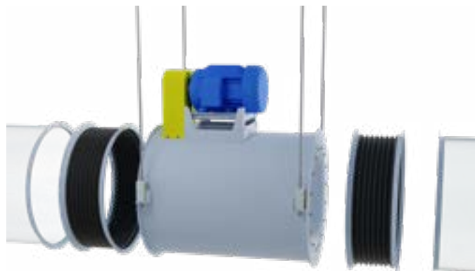
Ventilateurs hélico-centrifuges suspendus avec connecteurs de conduits flexibles
