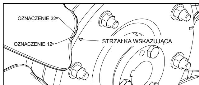
Rys. 12. Oznaczenia wskazujące kąt łopatki śmigła „E”
