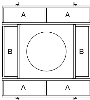
Fan Size 21
